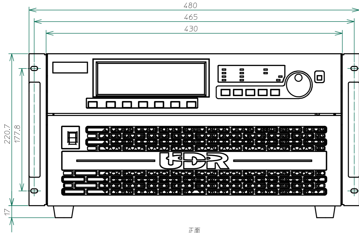
正面
