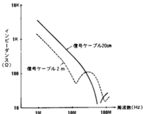
リップルメータ対地インピーダンスの例
