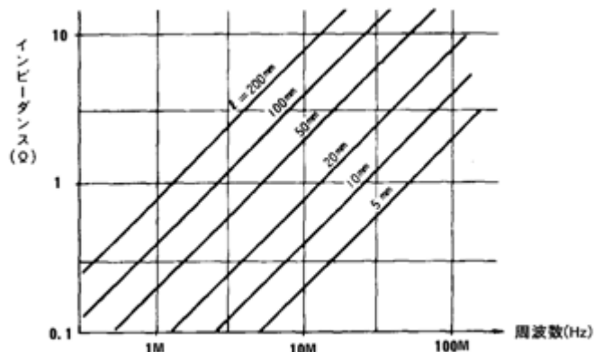
グランド線の長さインピーダンスの関係
