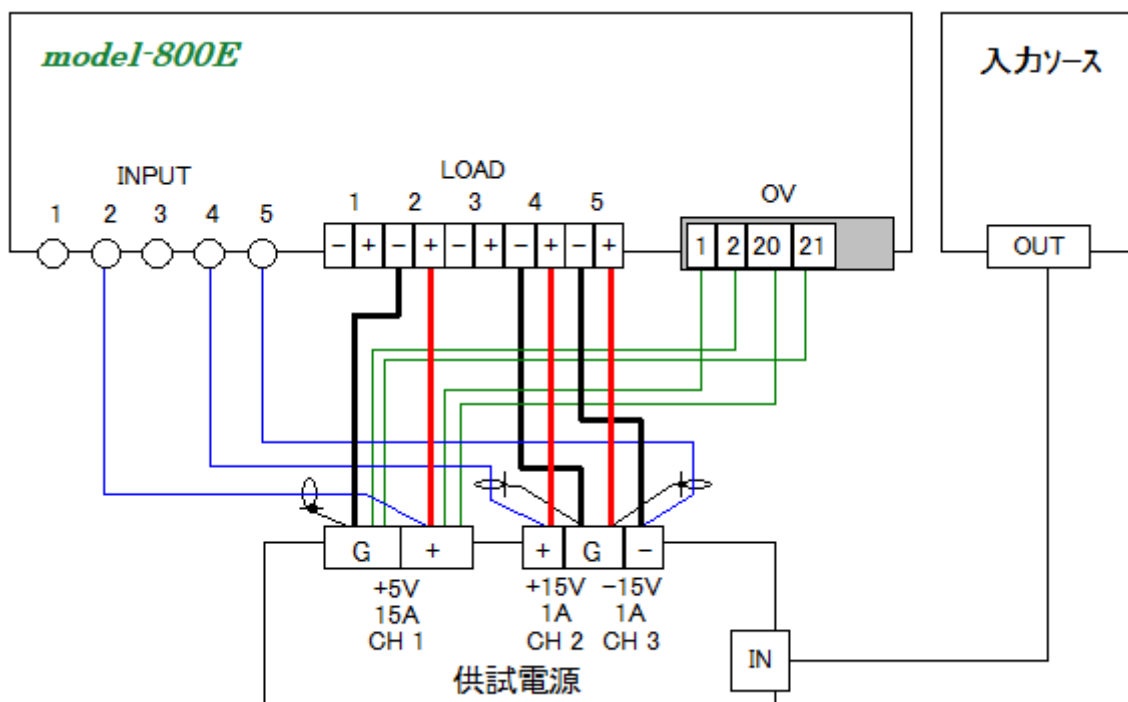
供試電源との接続例
