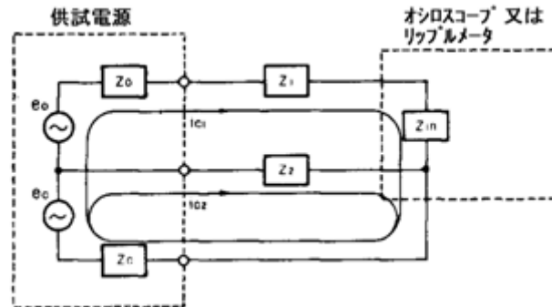
コモンモードノイズに対する等価回路
