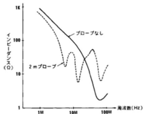
100 MHz オシロスコープの対地インピーダンスの例
