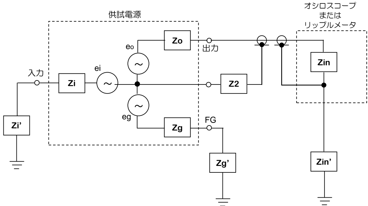
各端子ノイズ発生源と測定系の等価回路
