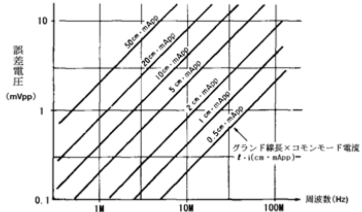
コモンモード誤差の早見表
