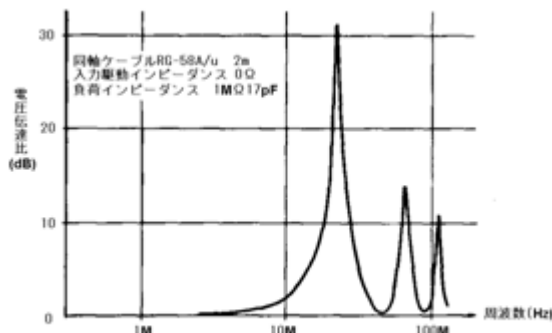
負荷開放時の同軸ケーブル電圧伝達比
