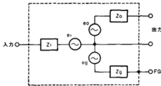
電源端子から見たノイズの発生源のモデル
