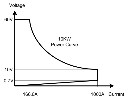
図 1-1.2 34110 負荷動作曲線 (1000A/60V)
