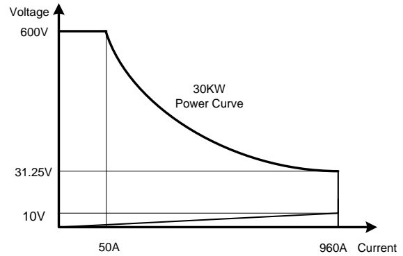
図 1-1. 12 34230 負荷動作曲線 (960A/600V)
