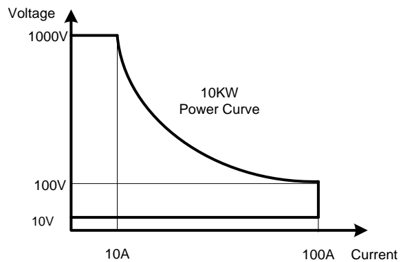
図 1-1. 14 34310 負荷動作曲線 (100A/1000V)
