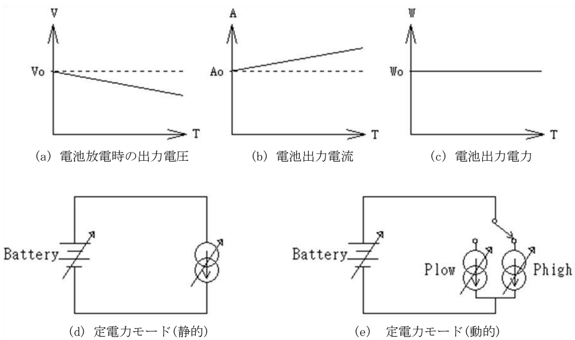
図 5-7: 定電力モード動作モードのアプリケーション
