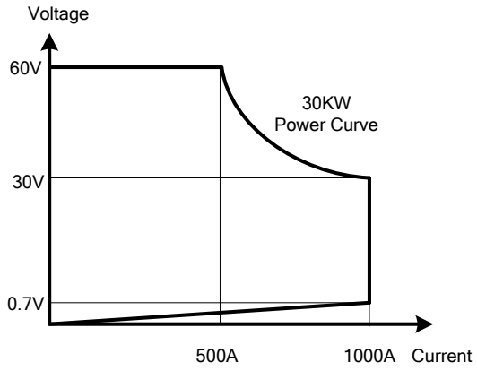
図 1-1.6 34130 負荷動作曲線 (1000A/60V)
