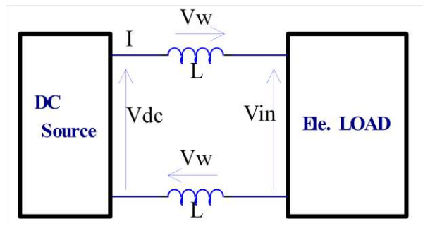
電源装置と負荷装置との接続図
