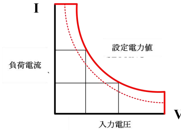
図 1-5 定電力モード特性図
