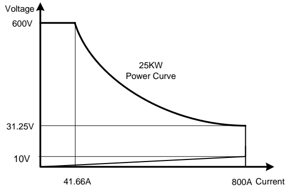
図 1-1. 11 34225 負荷動作曲線 (800A/600V)
