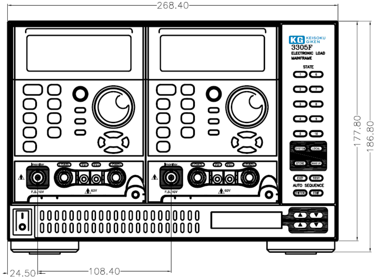
図3-1 3305Fフロントパネル
