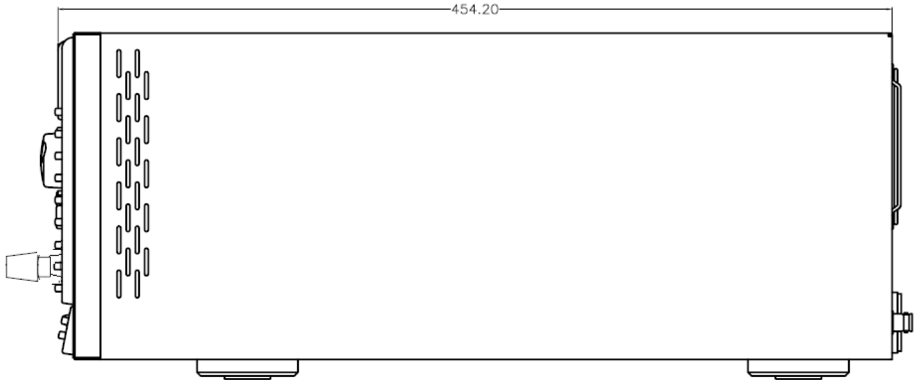
図3-2 3305Fサイドパネル
