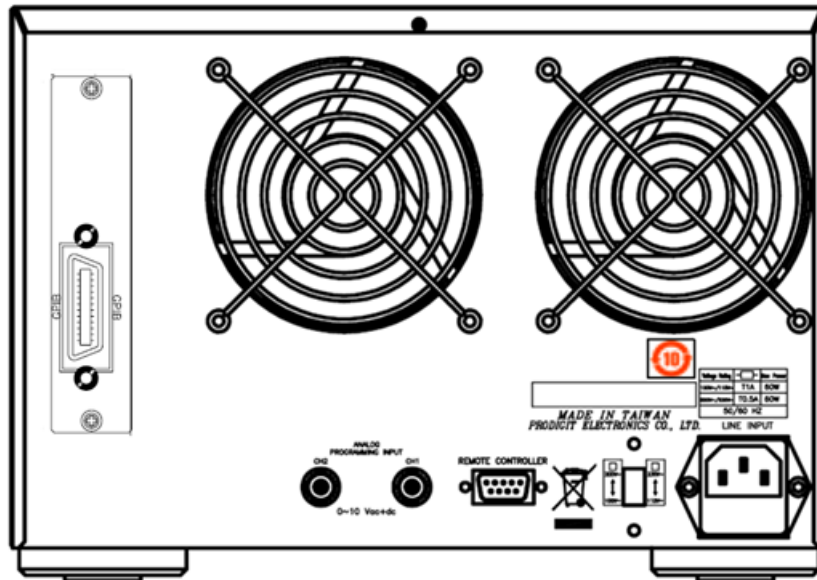
図3-3 3305F リアパネル
