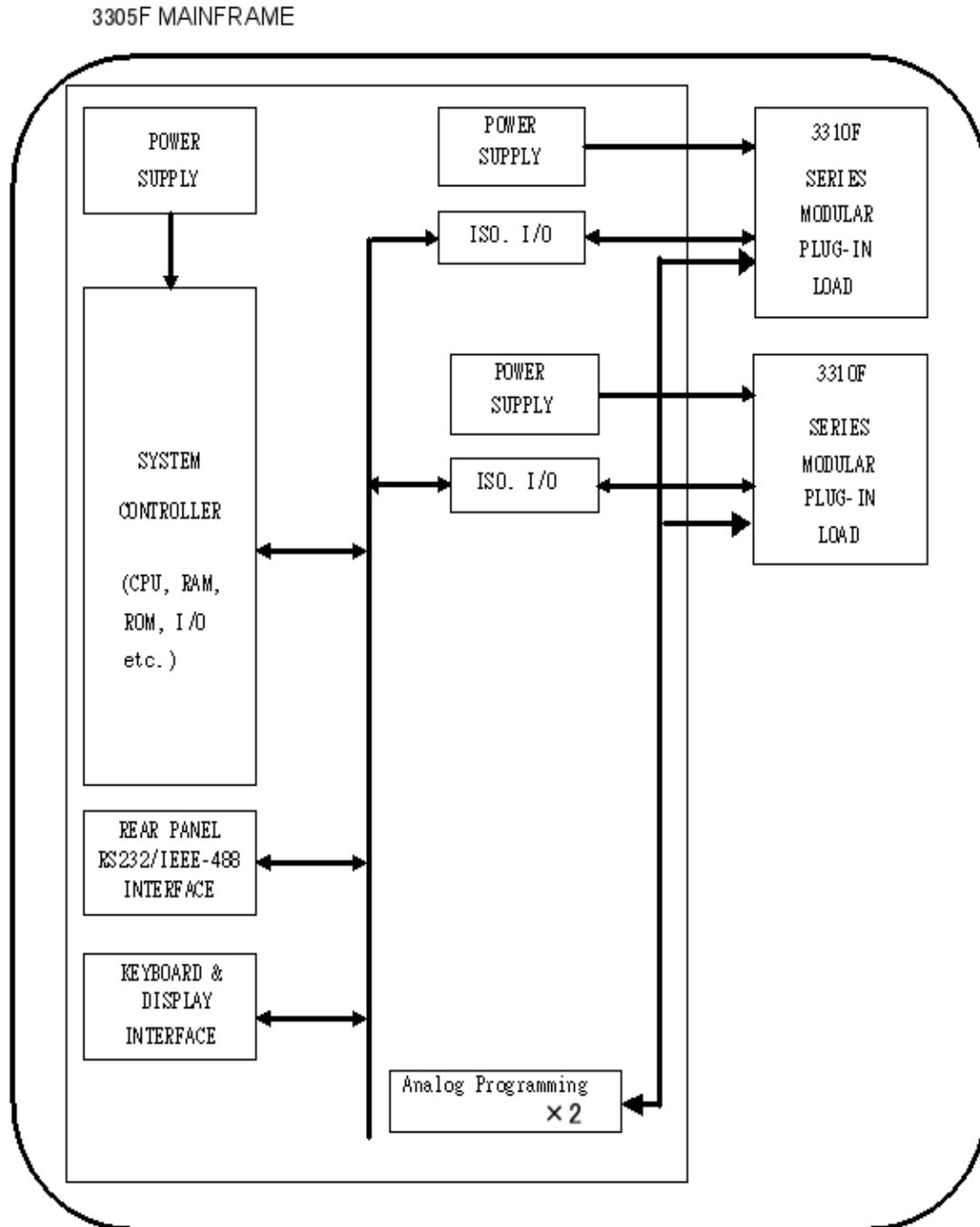
図1-1 3305F ブロックダイアグラム
