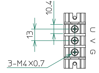
△ 出力端子台詳細
