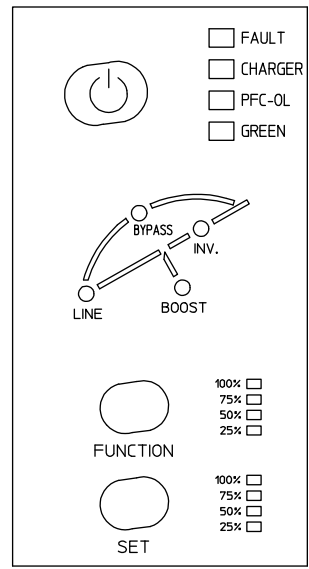
操作パネル詳細
