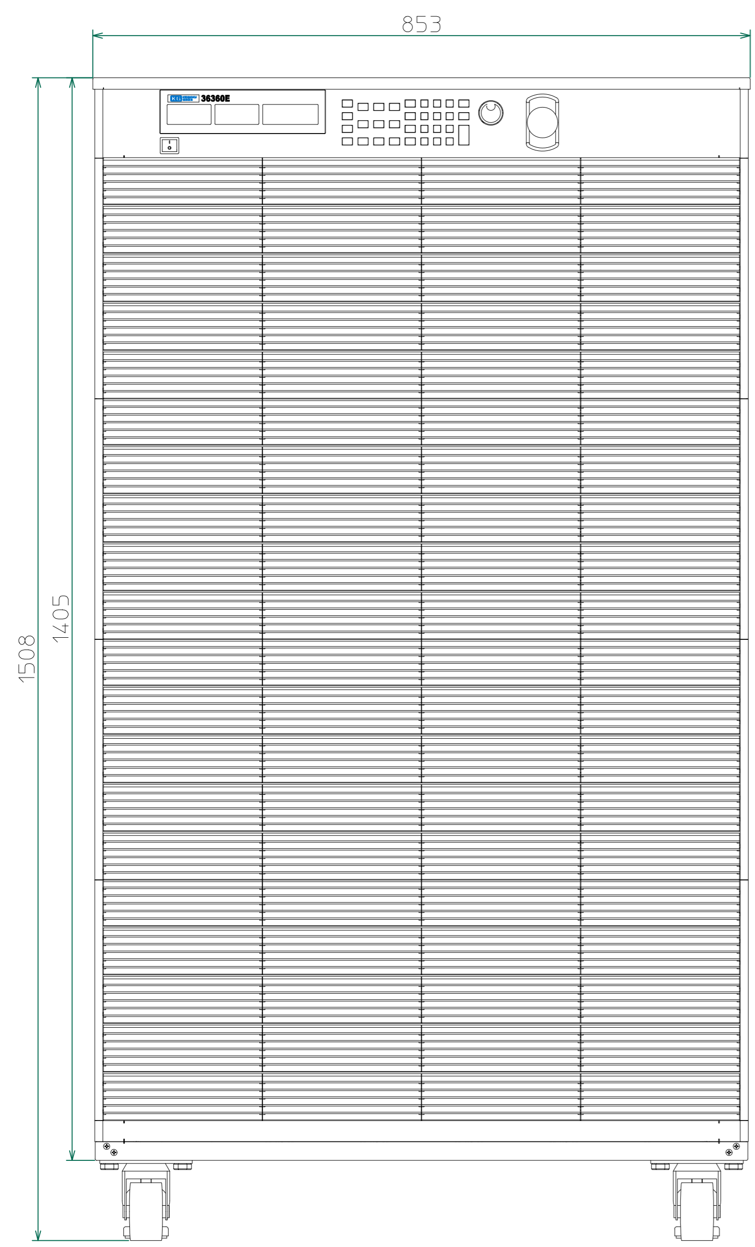
正面
