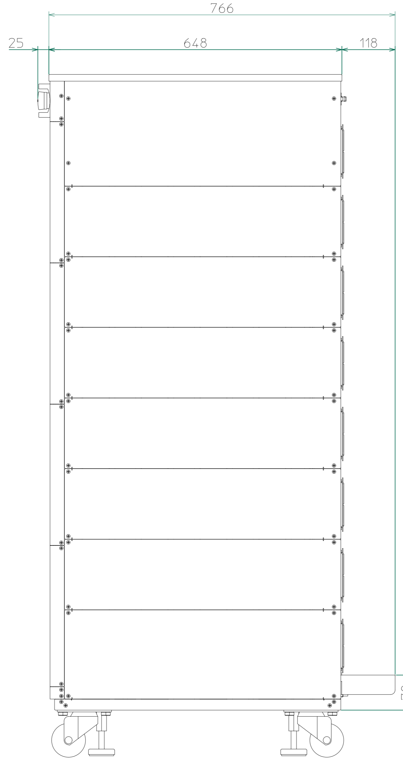
右側面
