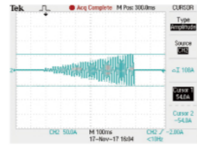
出力波形
