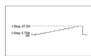
設定時波形
