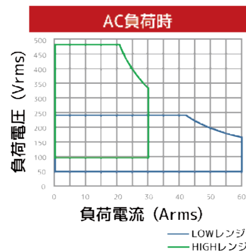
NT-AA-10KE-L(C) 負荷電力カーブ
