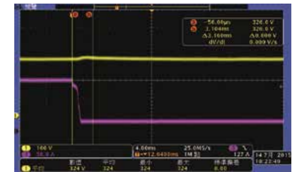
立ち下がり時の応答 3.16ms
