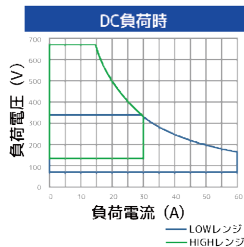
NT-AA-10KE-L(C) 負荷電力カーブ
