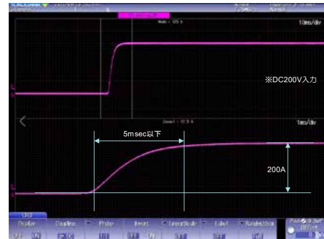
立上り電流波形(DC200V入力200A時)
