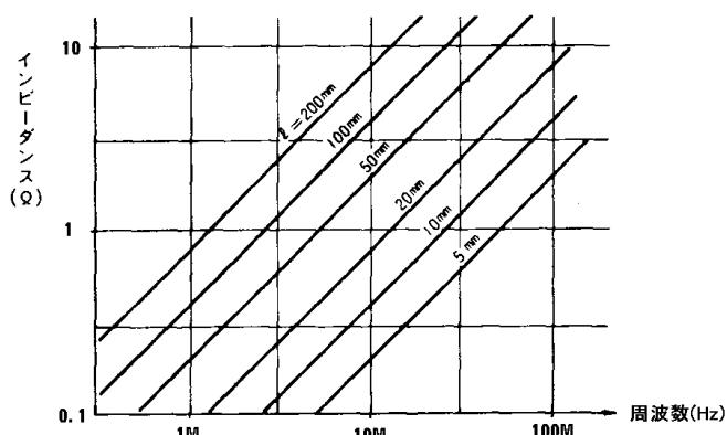
図9-5 グランド線の長さとのインピーダンスの関係
