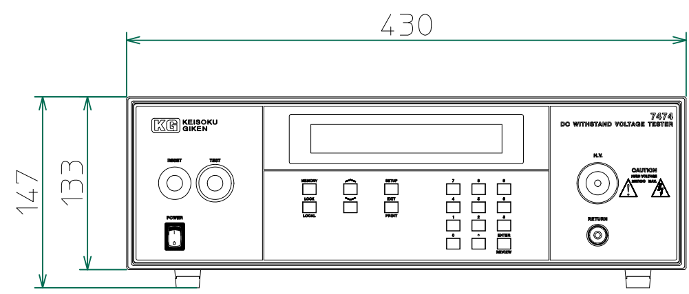
正面
