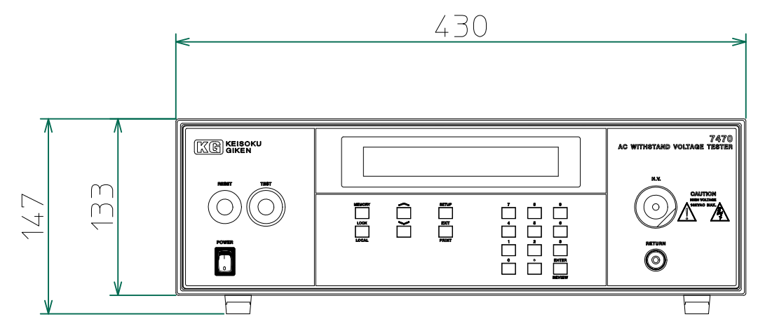
正面
