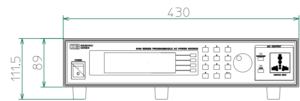
正面
