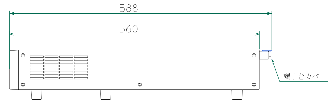
右側面
