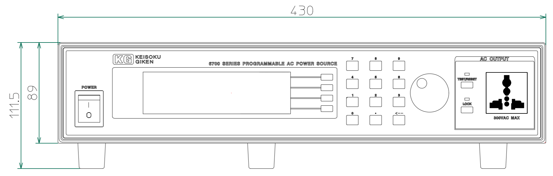
正面
