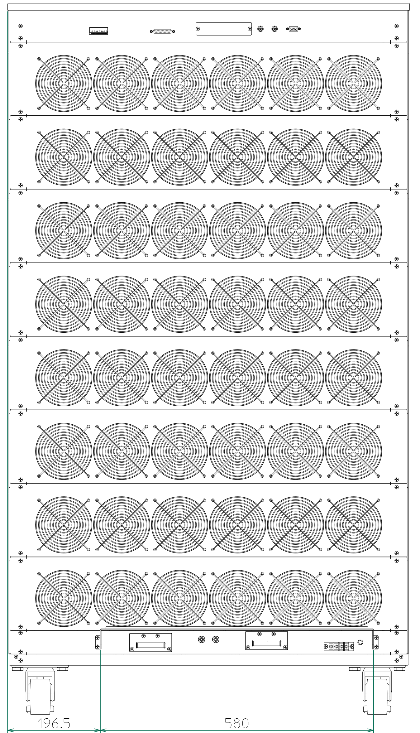
背面
