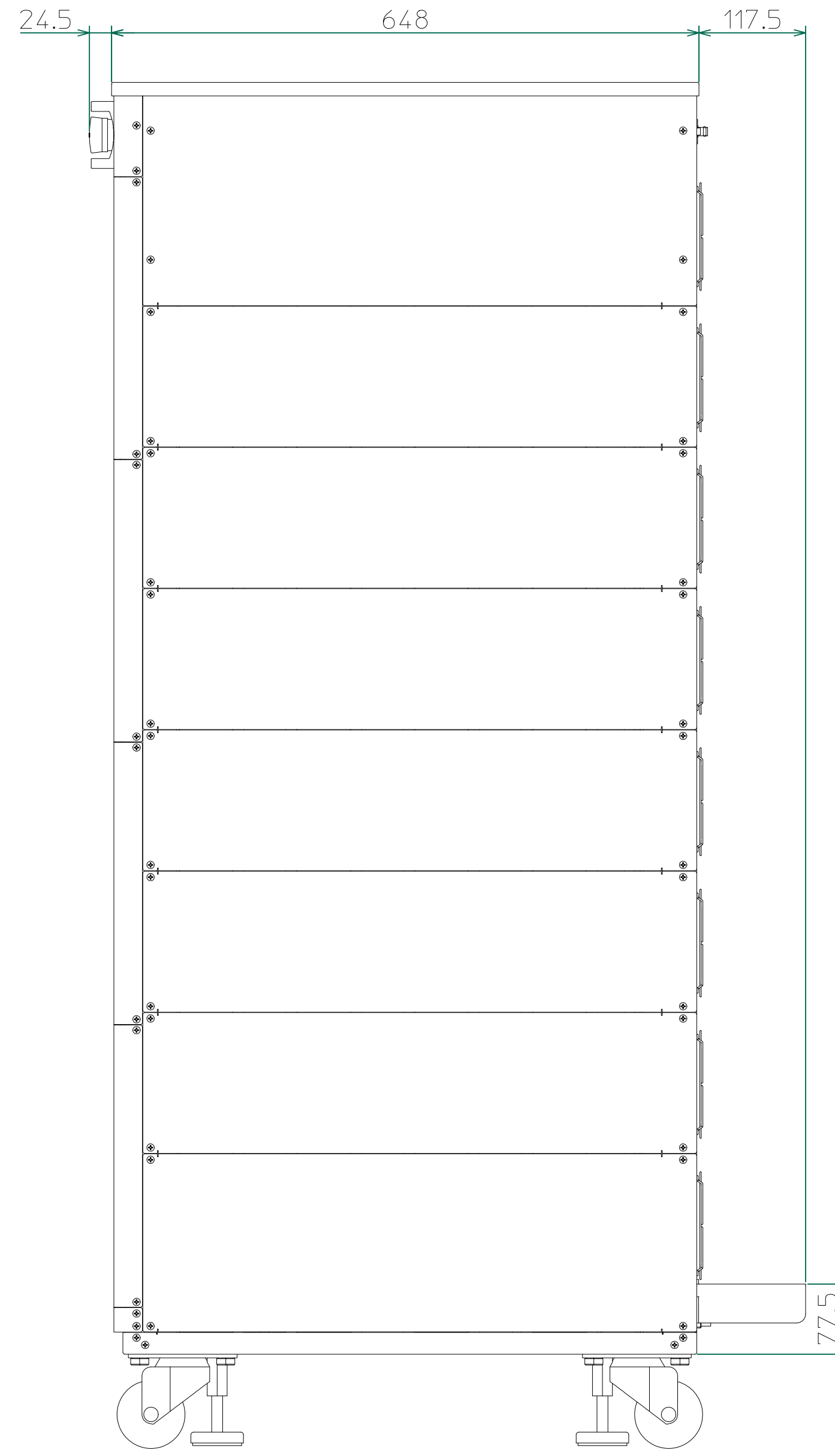
右側面
