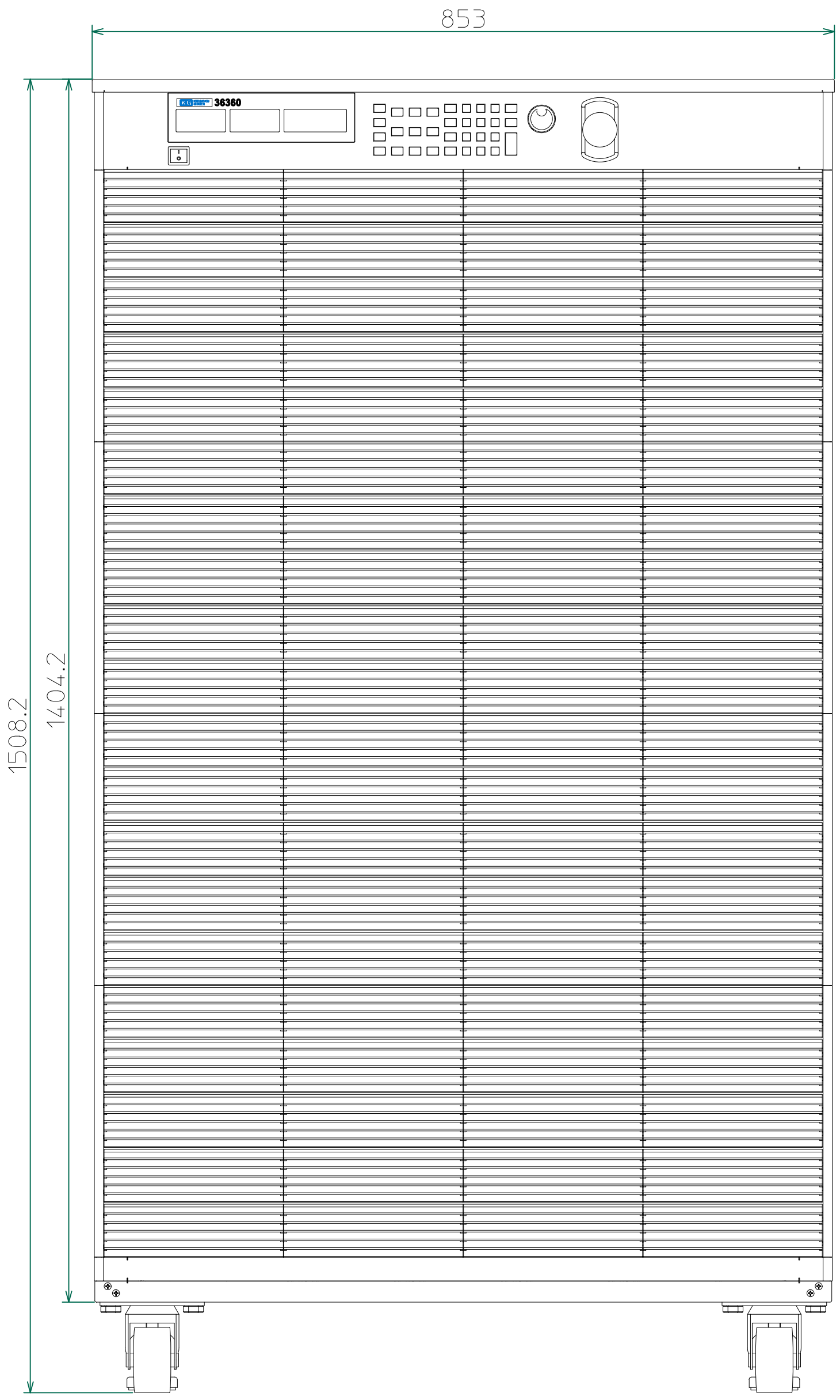
正面
