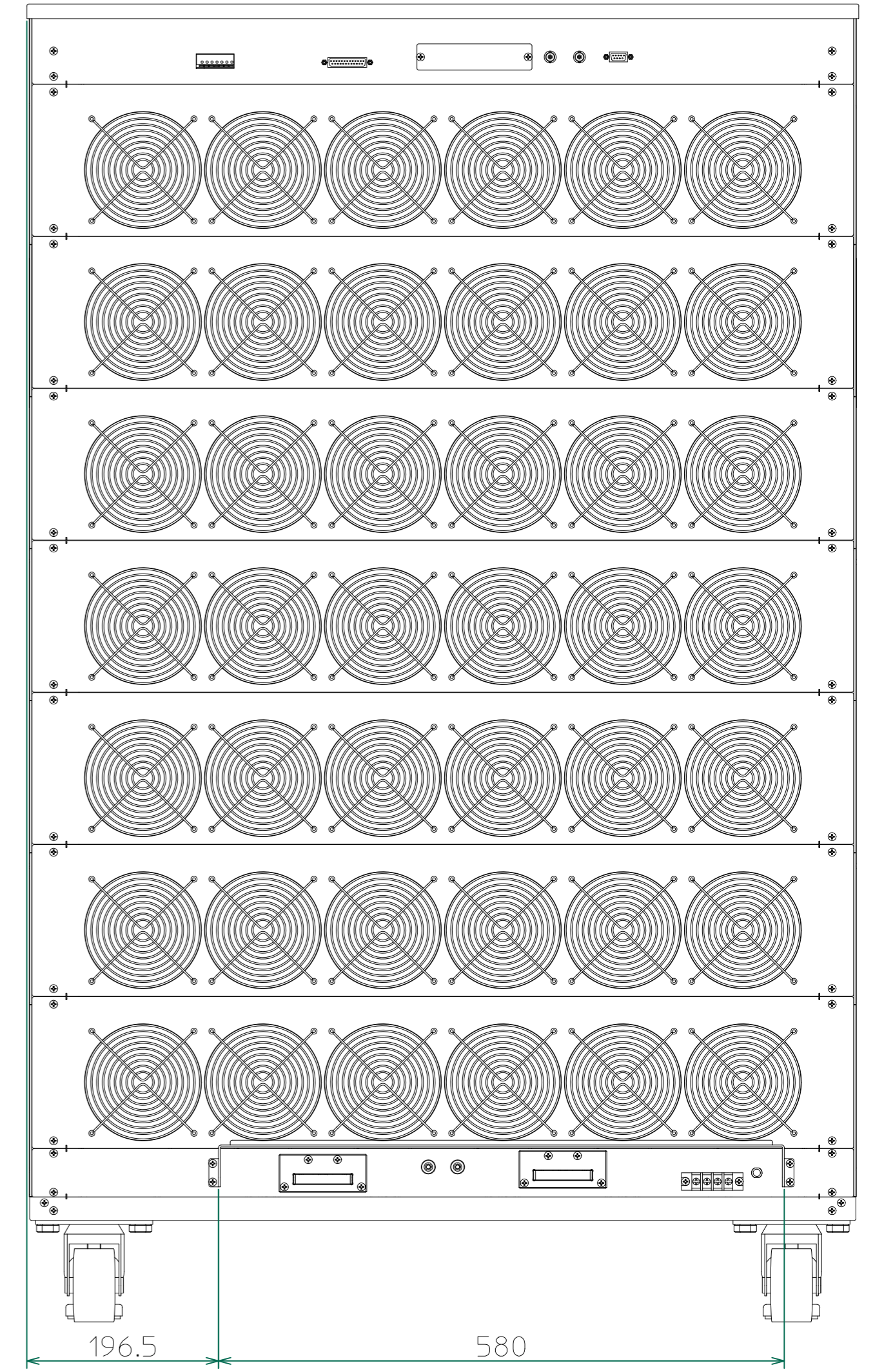
背面
