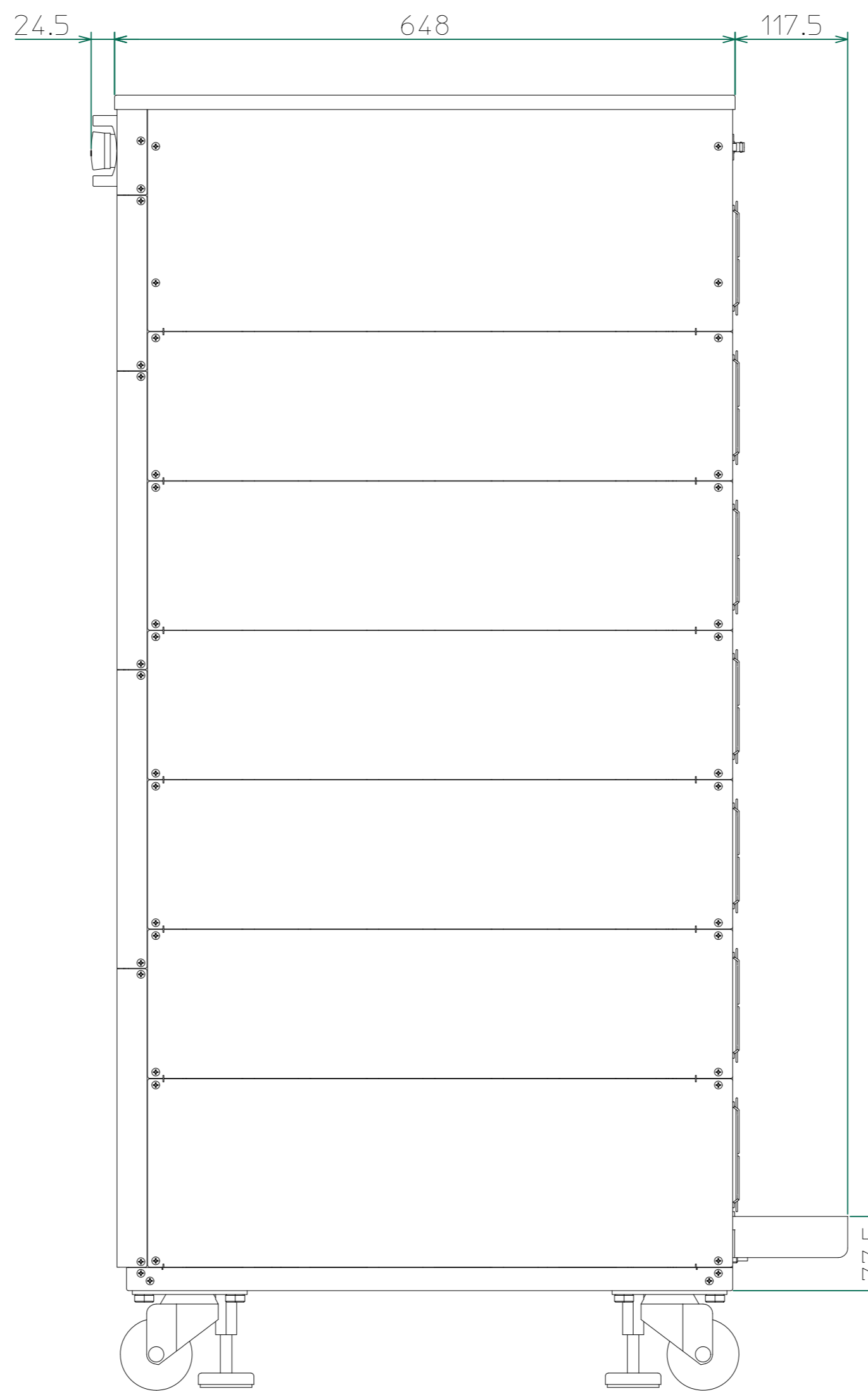
右側面
