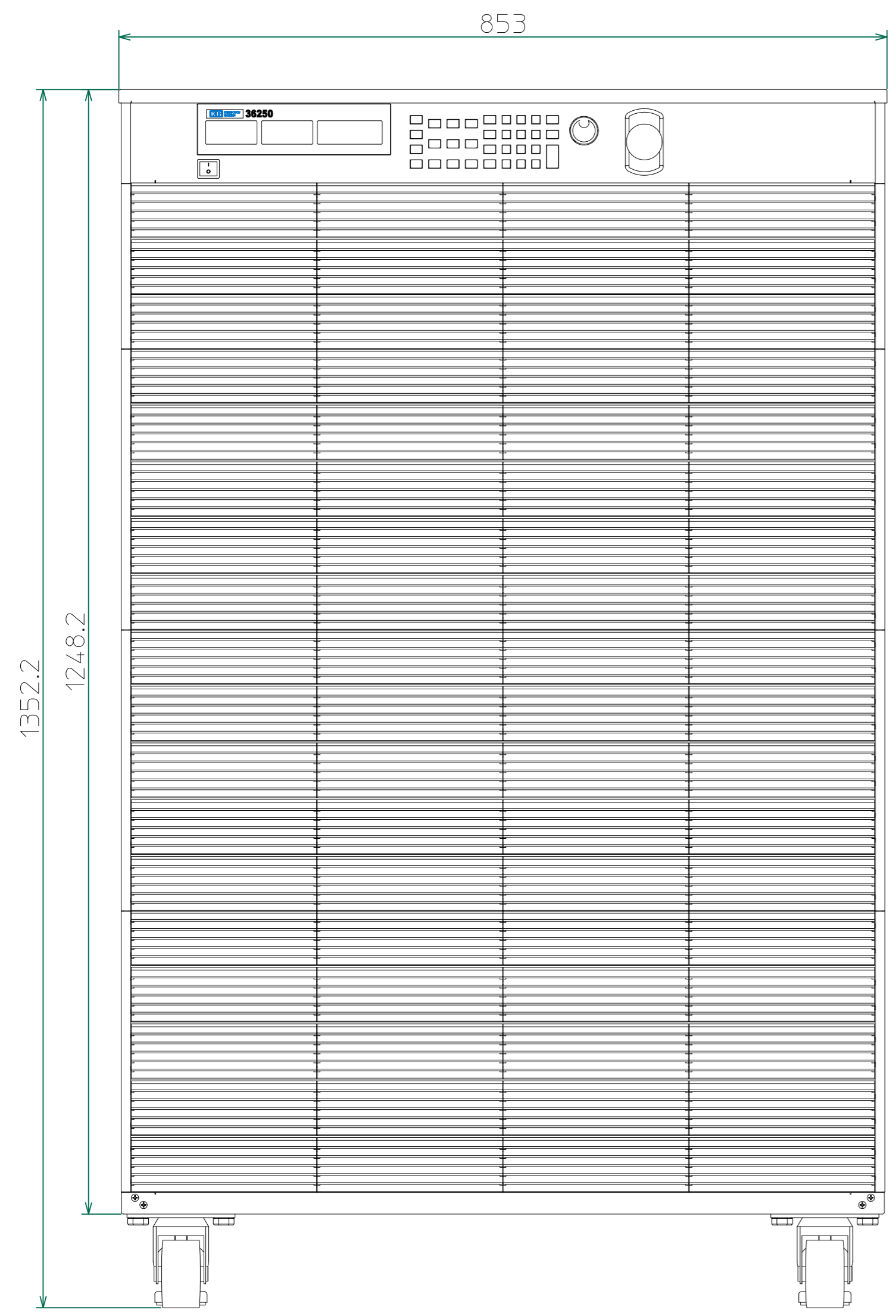
正面
