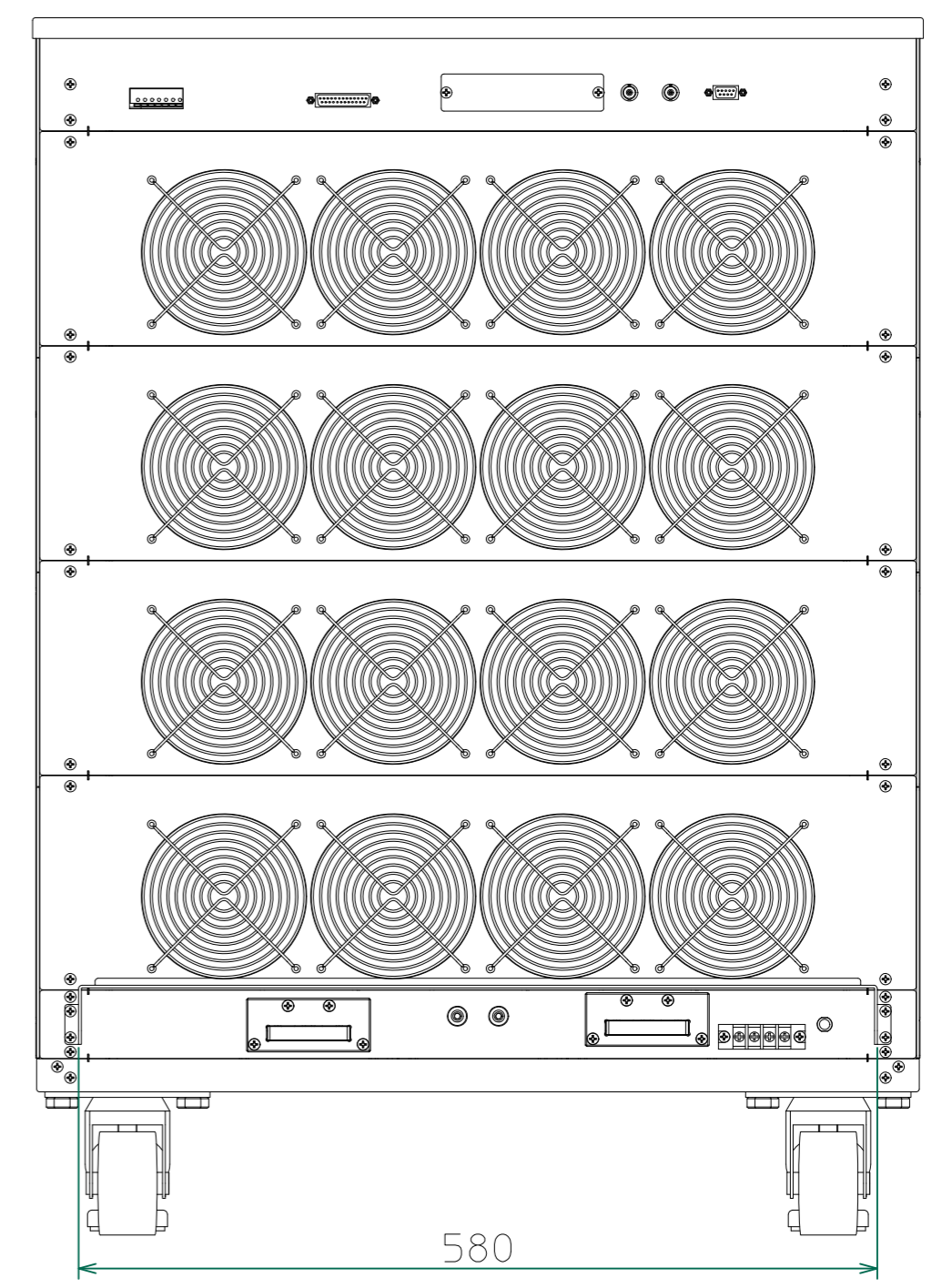
背面
