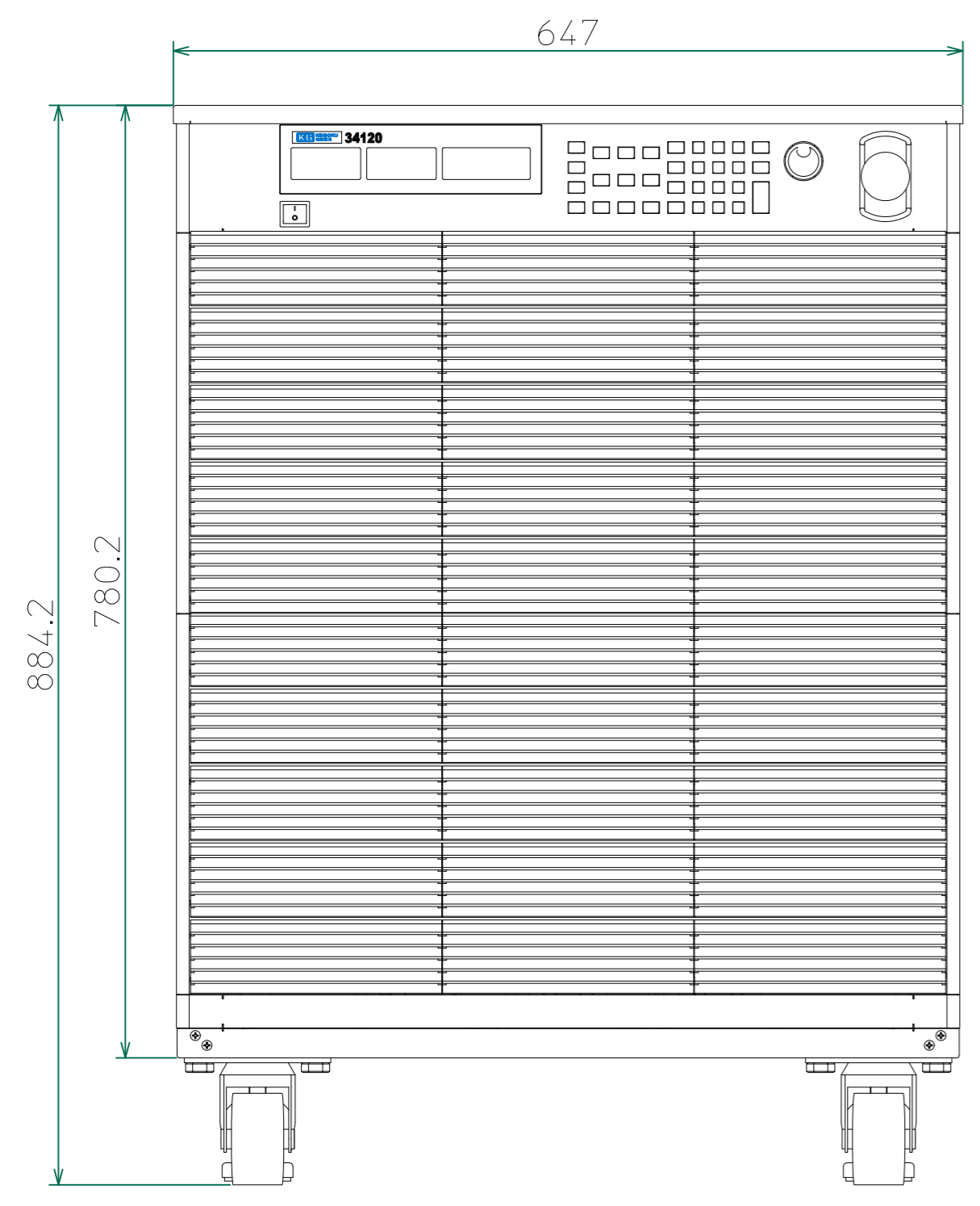
正面
