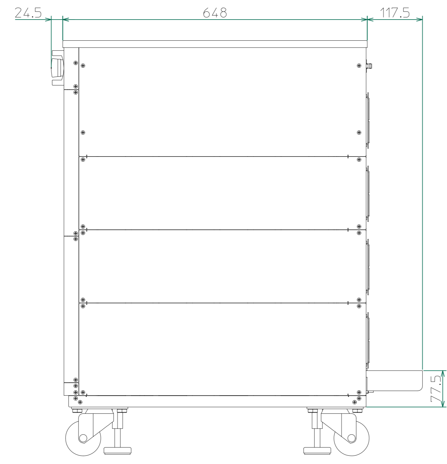
右側面
