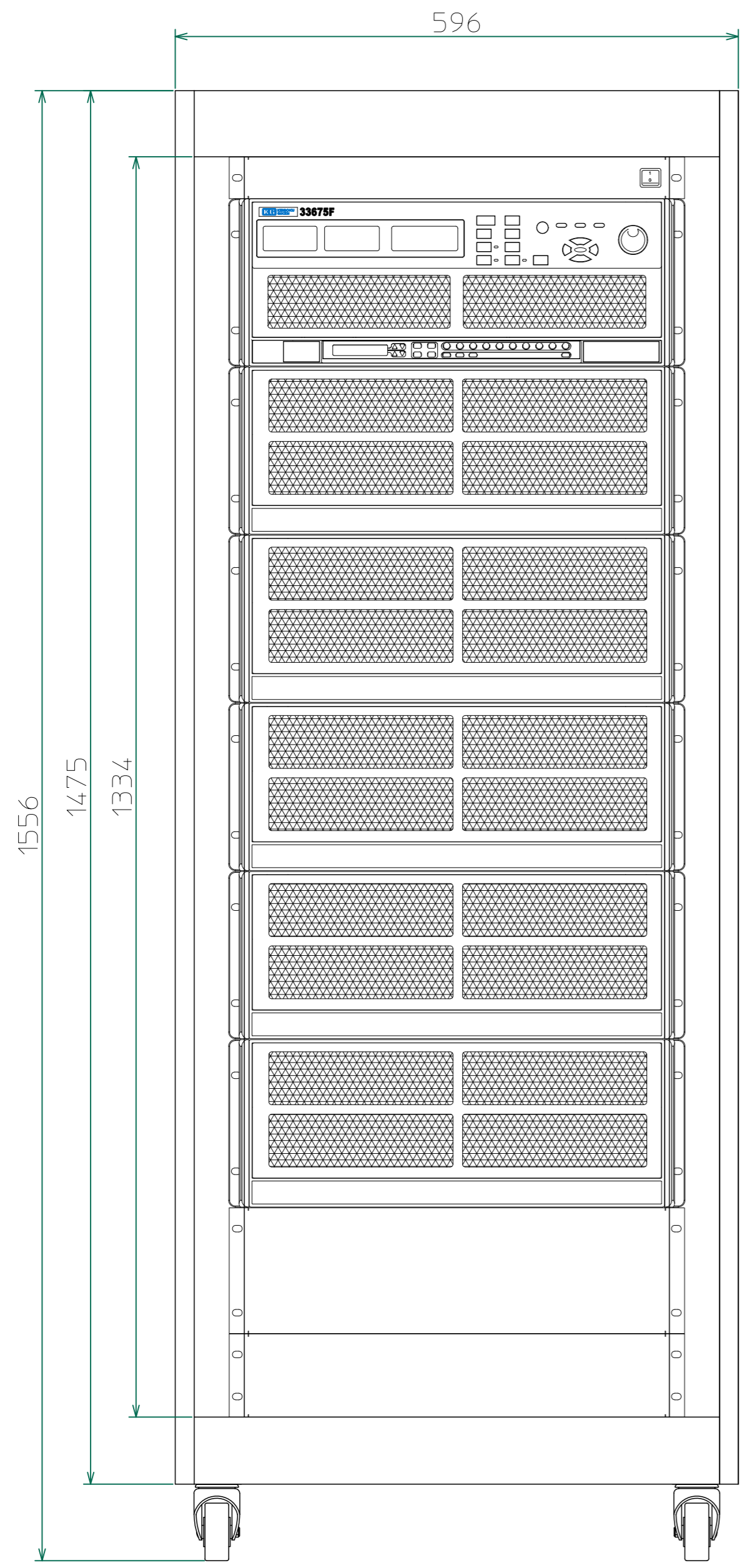
正面
