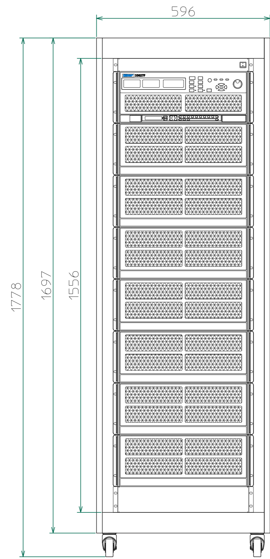
正面
