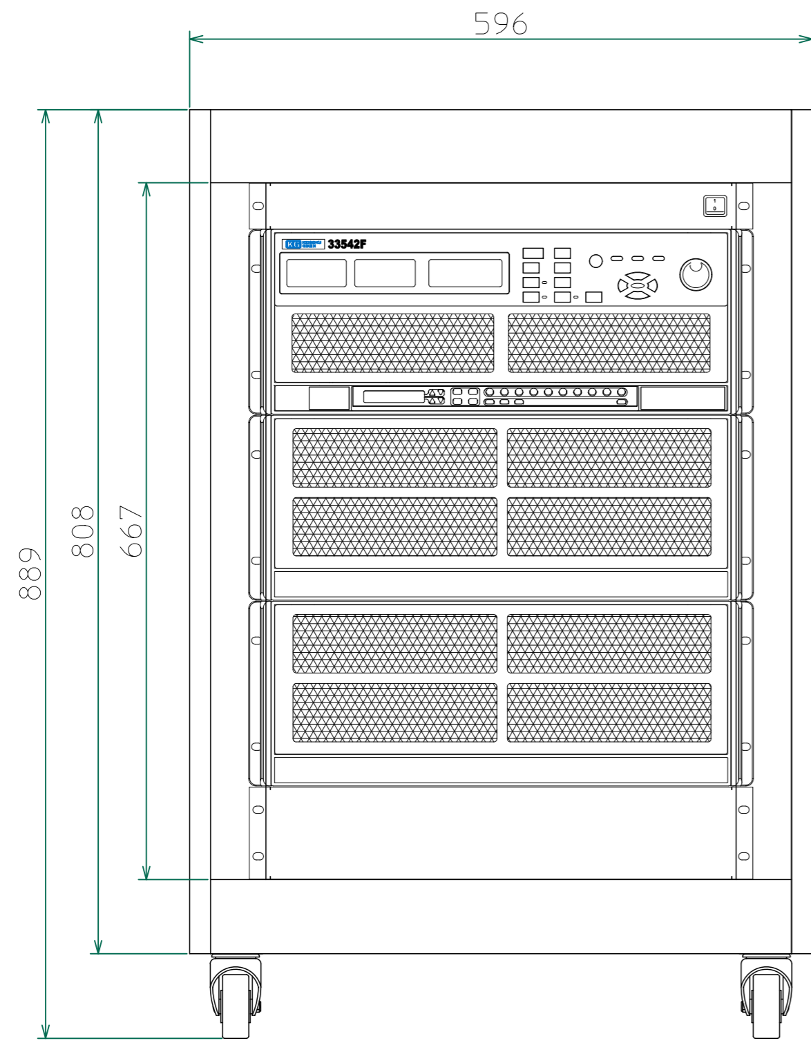
正面
