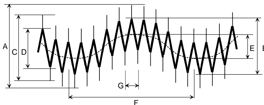
スイッチング電源の出力電圧例
