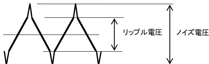
スイッチングリップル波形例
