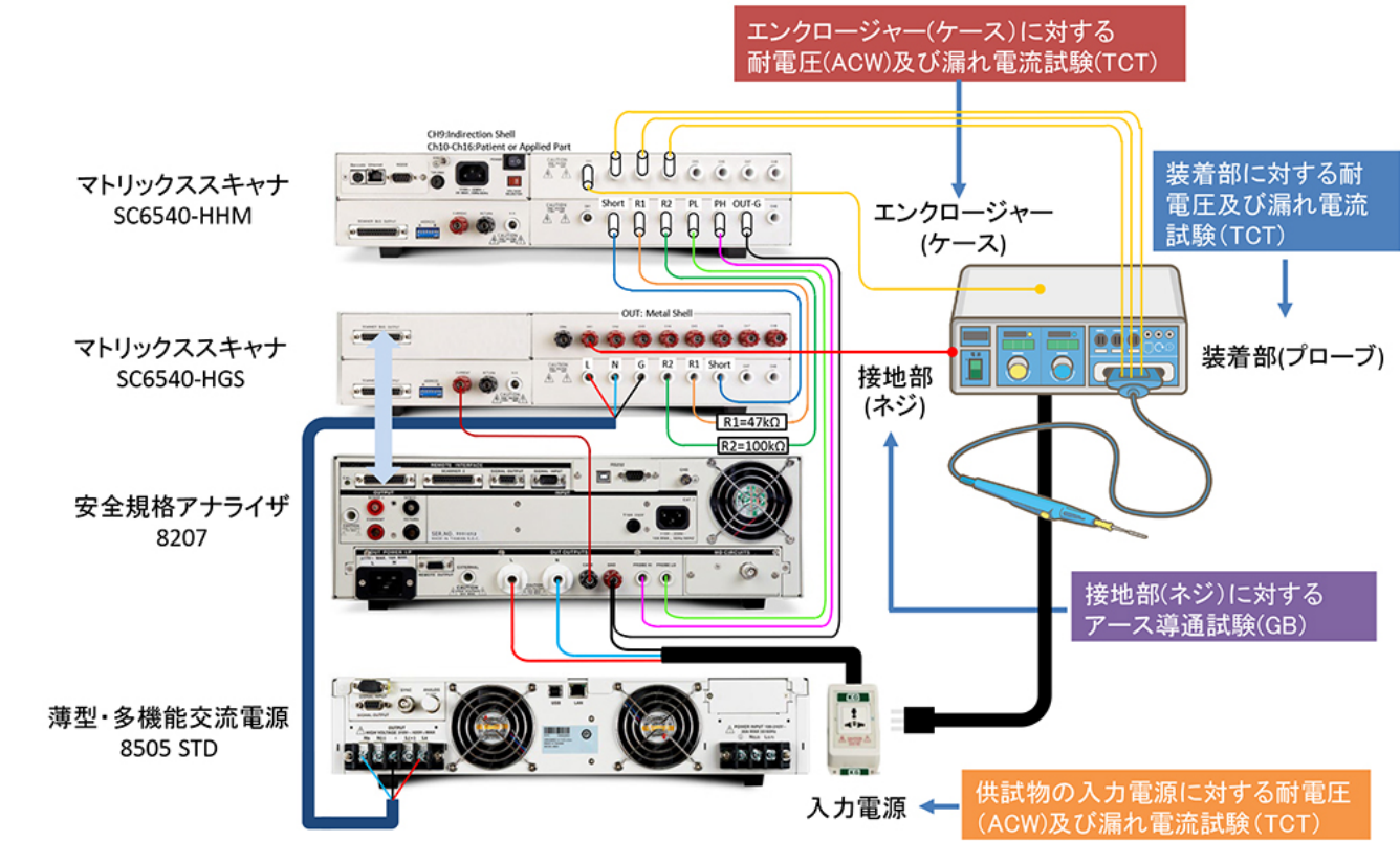
電気メスシステムの安全規格試験接続方法例
