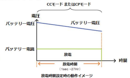
指定時間までCC/CP放電
