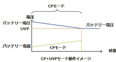
指定電圧までCP放電
