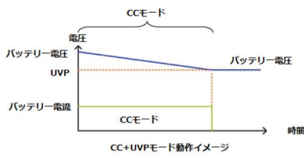
指定電圧までCC放電
