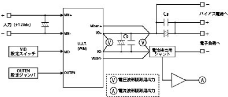
テストフィクスチャ回路構成図
