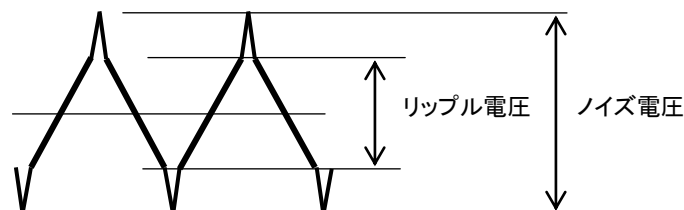
図 B.2 スwitchングリップル波形例
