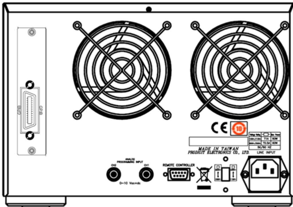
図3-3 3305F リアパネル
